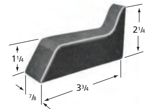
»»» ATI752F-1 1.25 LBS
