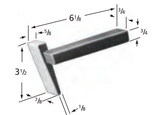
»»» ATI752Z-1 1.50 LBS
