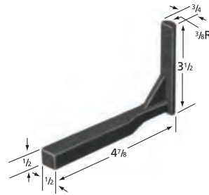
»»» ATI751V-1 1.25 LBS
