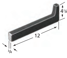
ATI625 5.25 LBS
