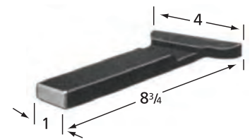
ATI632 4.50 LBS
