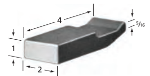
ATI637 1.75 LBS
