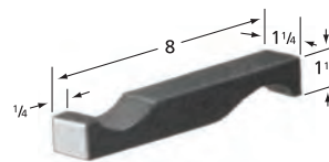
»»» ATI752C-1 2.50 LBS
